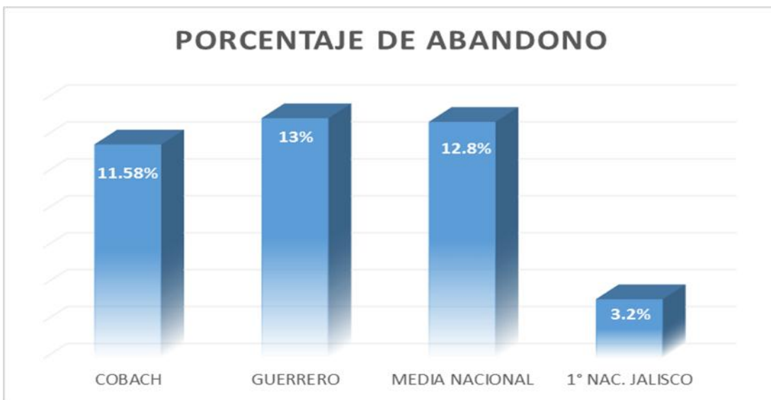
Gráfica 2. Análisis comparativo del abandono a nivel nacional.
