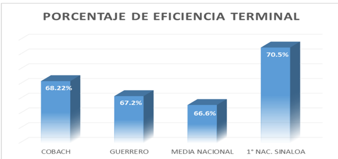
Gráfica 3. Comparativo de la Eficiencia Terminal a nivel nacional. 2
